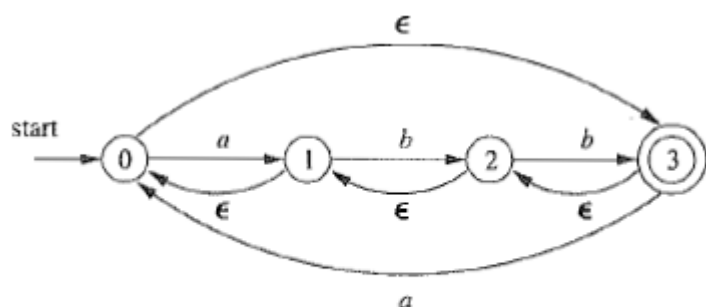
图 3-30 练习 3.6.4 的 NFA
