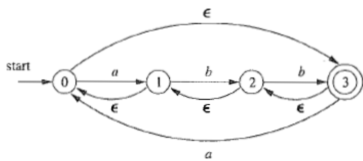
图 3-30 练习 3.6.4 的 NFA
