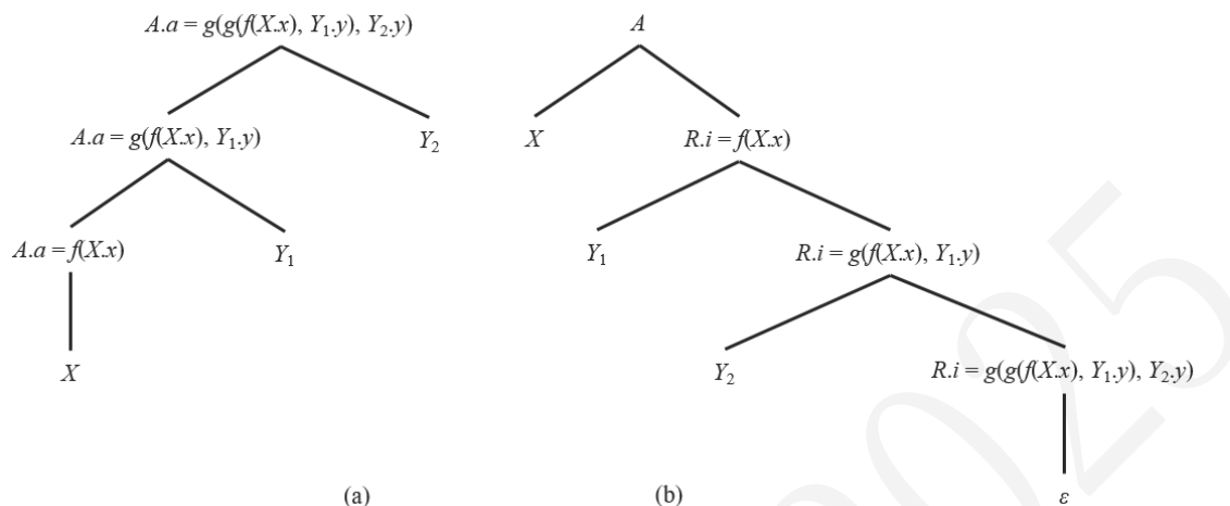
图 3.3 消除一个后缀 SDT 中的左递归
