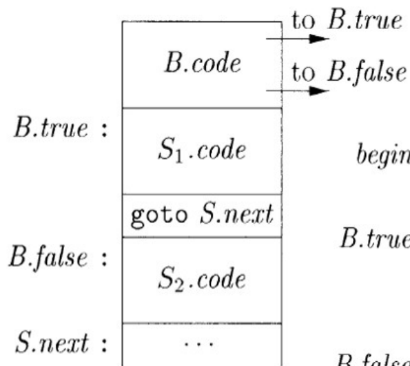
b) if-else
