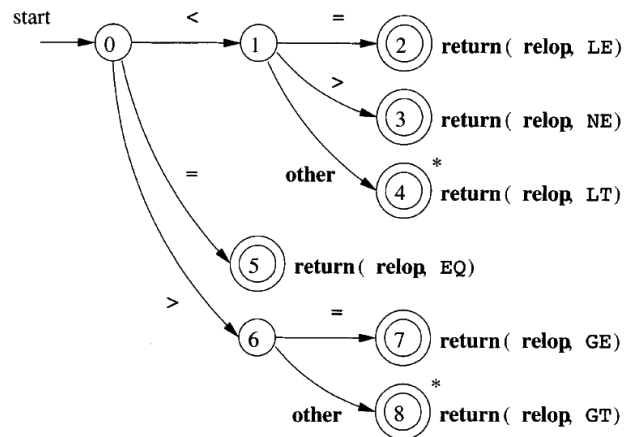
图 3-13 词法单元 relop 的状态转换图
